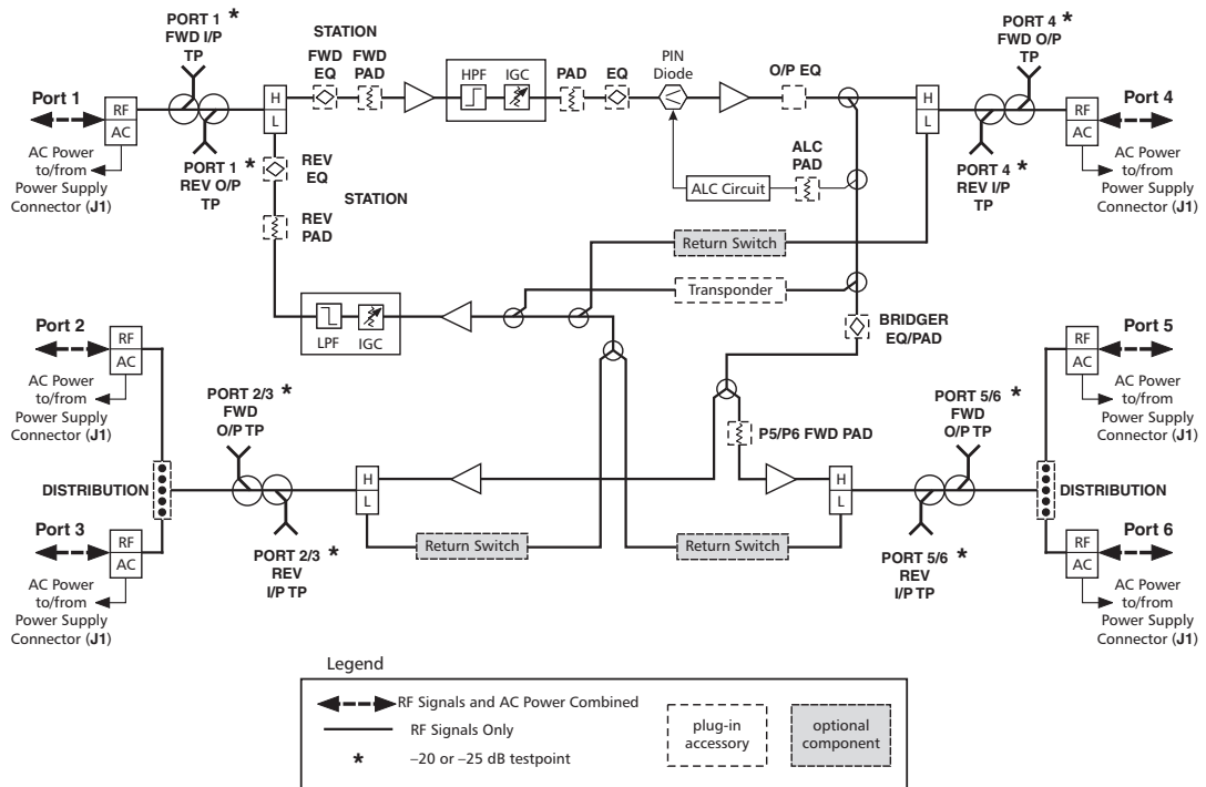
Flex Max901e Trunk Amplifier
